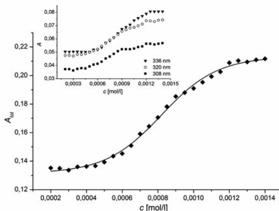
Graf 1. Závislosť súčtu absorbií hlavných pyrénových píkov ( A_{tot} ) od koncentrácie ( c ) látky XXIX Z vo vodnom prostredí pri 25 °C
