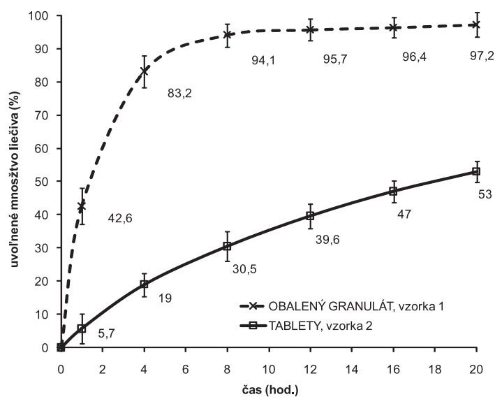
Obr. 1. Liberačné profily metoprololiumsukcinátu z obaleného granulátu a z matricových tabliet. 100 mg Eudragit® NE 30 D
