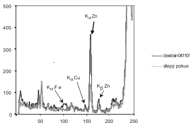
Obr. 2. Spektrum žiarenia zdroja ^{238}\text{Pu} po interakcii s filtrom – dextrans A a čistým filtrom
