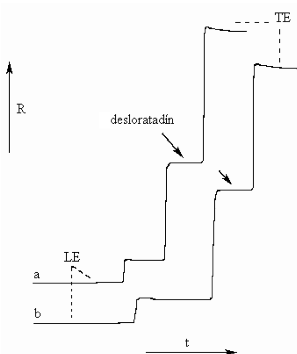
Obr. 2. Izotachoforeogramy vodných roztokov dvoch liekových foriem desloratadínu: Aerius obalované tablety (a) a Aerius sirup (b) v elektrolytovom systéme č. 2
